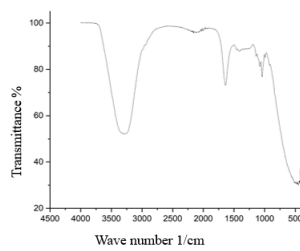
Fig.1. BRIX3000 IR spectrum.
